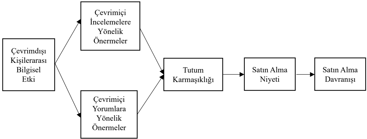
Şekil 1. Araştırma Modeli
