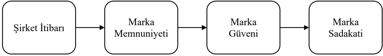
Şekil 1. Araştırma Modeli
