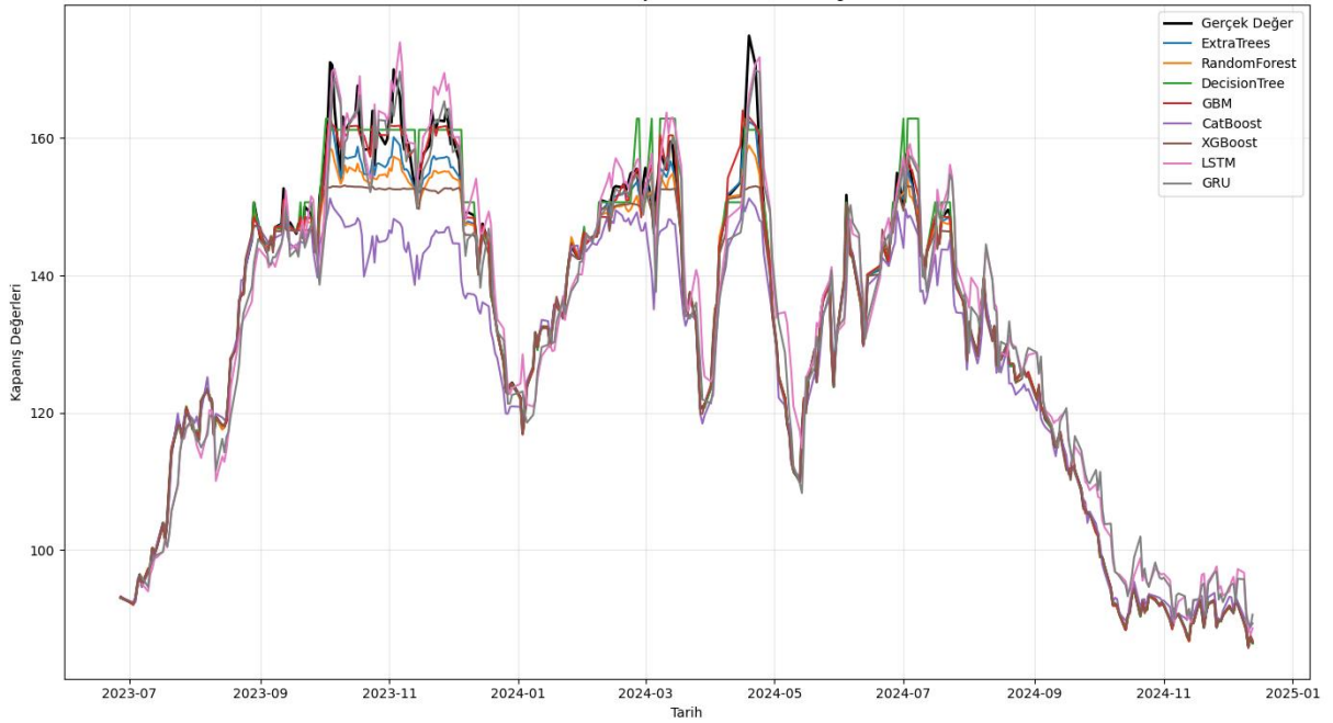
Görsel 1. Tüm Modellerin Gerçek ve Tahmin Edilen Değerleri
