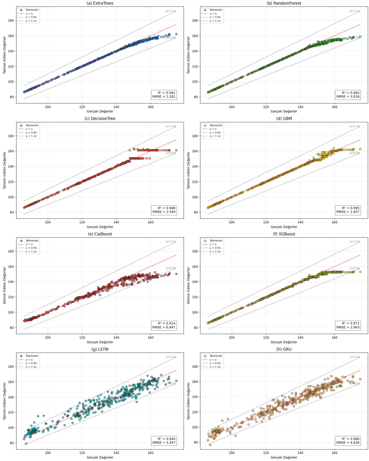
Görsel 4. Modellerin Gerçek ve Tahmin Edilen Değerler Arasındaki Dağılımı
