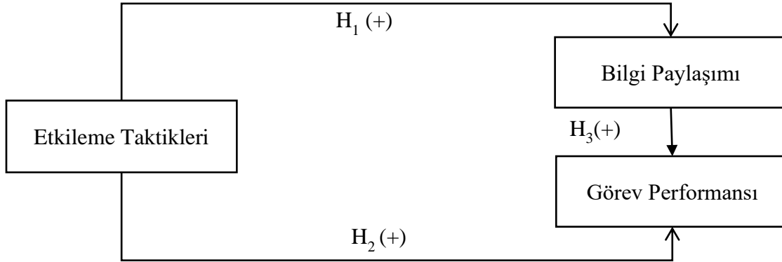
Şekil 1. Araştırmanın Modeli
