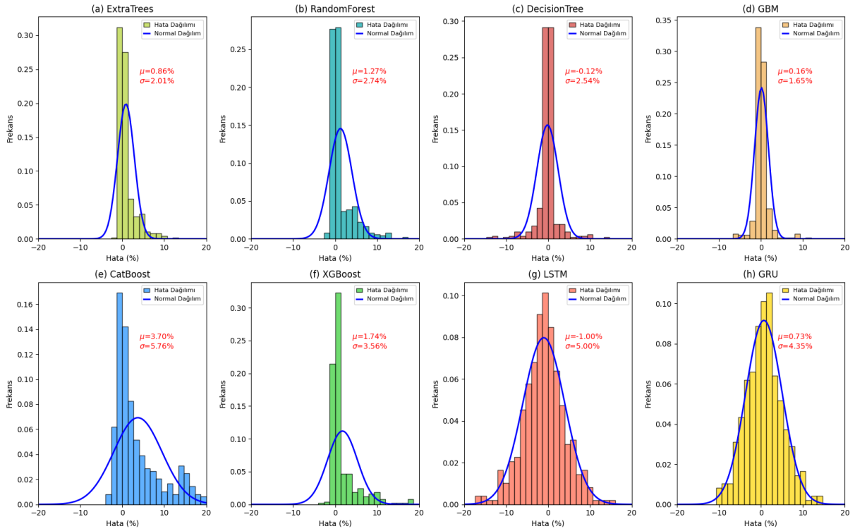
Görsel 3. Modellerin Hata Dağılımı ve Normal Dağılım Karşılaştırması
