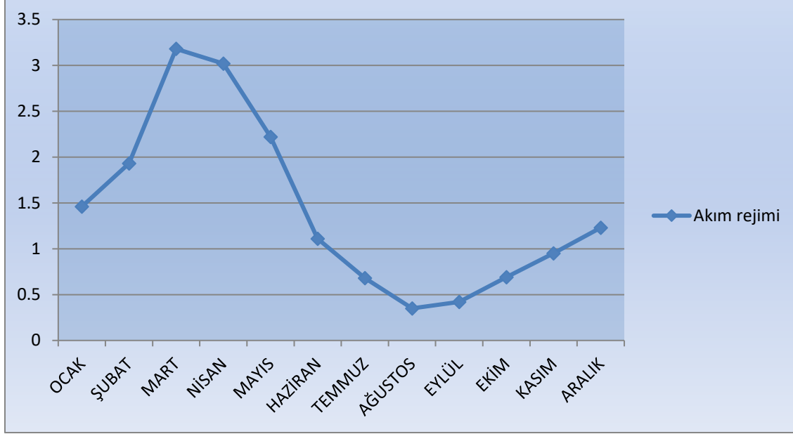
Şekil 3. Kürtün Çayı akım rejimi.
