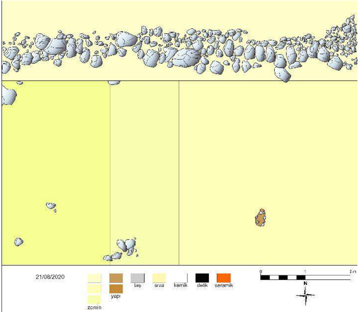
Görsel 2. C 3 plankaresi çizimi
