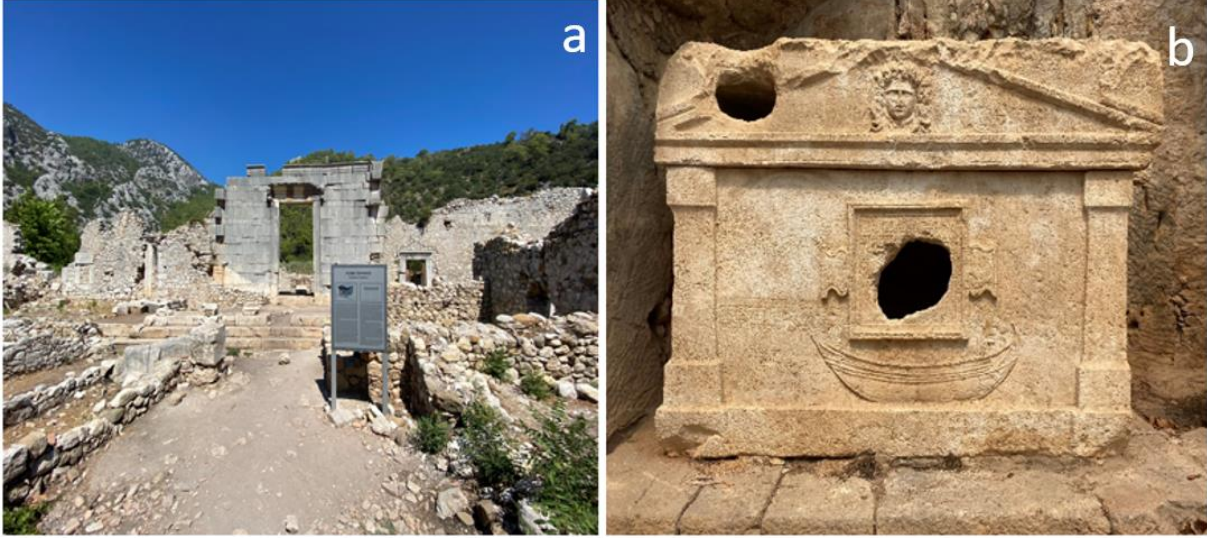
Foto 2a. Olympos Antik Kenti'nde Roma Tapınağı, b. Kaptan Eudemos'un Lahdi
