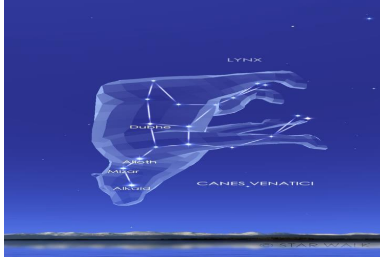
Görsel 6: Büyükayı Takımyıldızı
